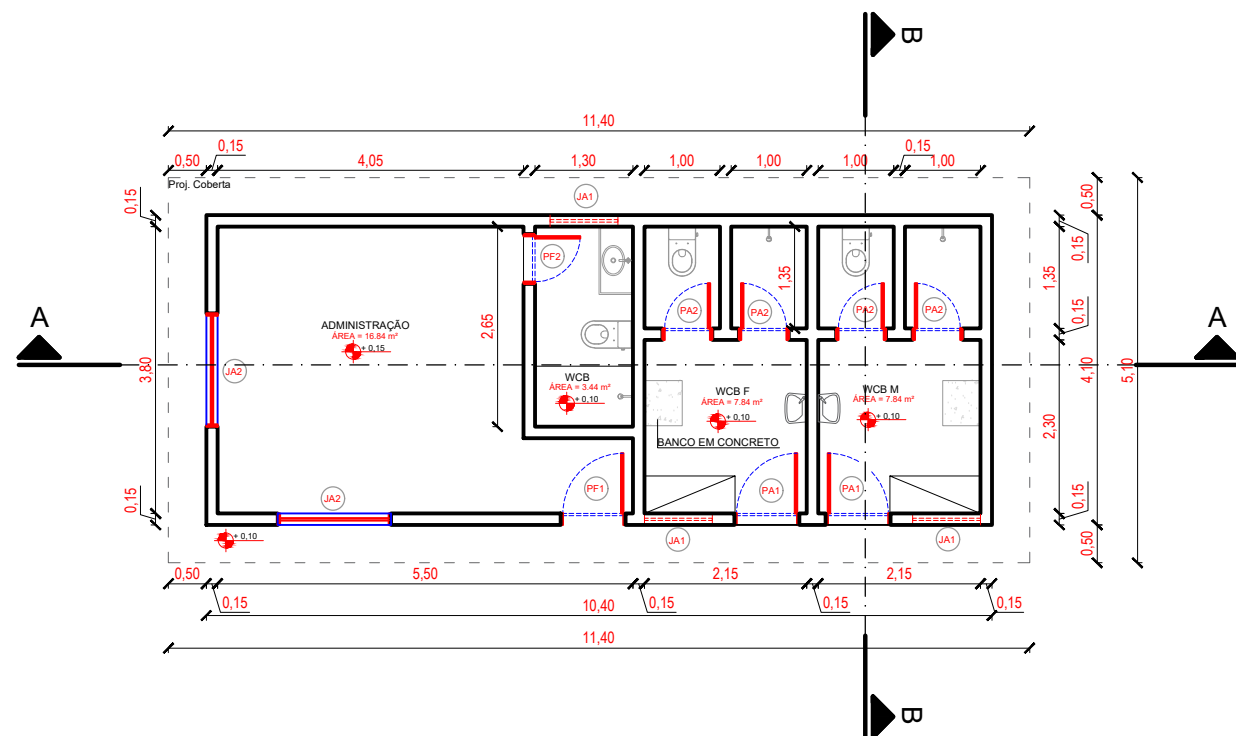
PLANTA BAIXA _ ADMINISTRAÇÃO ESCALA 1/100
