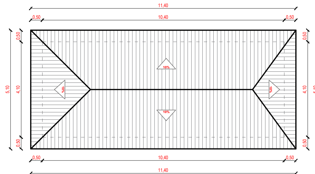
PLANTA DE COBERTA ESCALA 1/100
